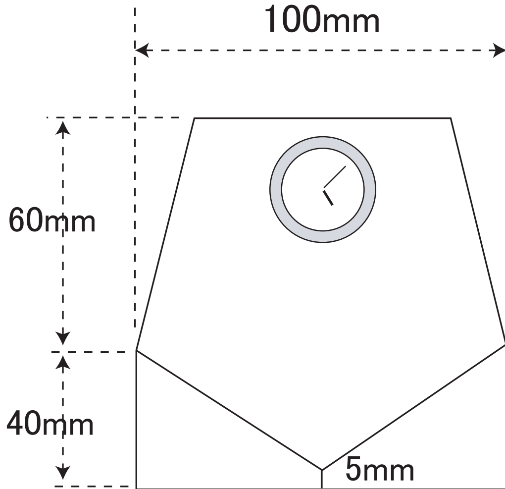
正面図
